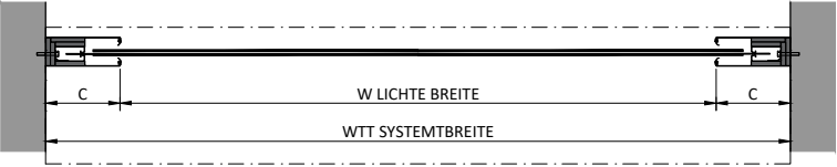
GEBÄUDEPLAN - MONTAGE IN DER ÖFFNUNG (LAIBUNGSMONTAGE)
