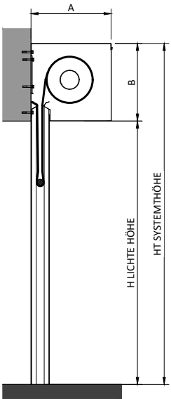
SCHNITT WANDMONTAGE
