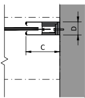
LAIBUNGSMONTAGE
