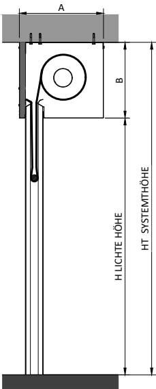
SCHNITT LAIBUNGSMONTAGE
